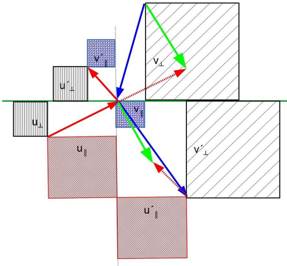
Abbildung 3: Impuls- und Energieerhaltung werden durch den Satz von Pythagoras einfach überprüfbar (schwarz Stoßachse und auf Planckobjekten erhaltene orthogonale Komponenten, rot von u , blau von v , grün erhaltene Relativgeschwindigkeit => Impuls). Das gilt bei jedem elementaren Ereignis, also Stoß. Die Summe der Geschwindigkeitsbeträge ändert sich aber.
